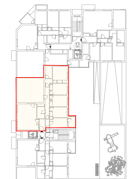
PLANTA ÁTICO
