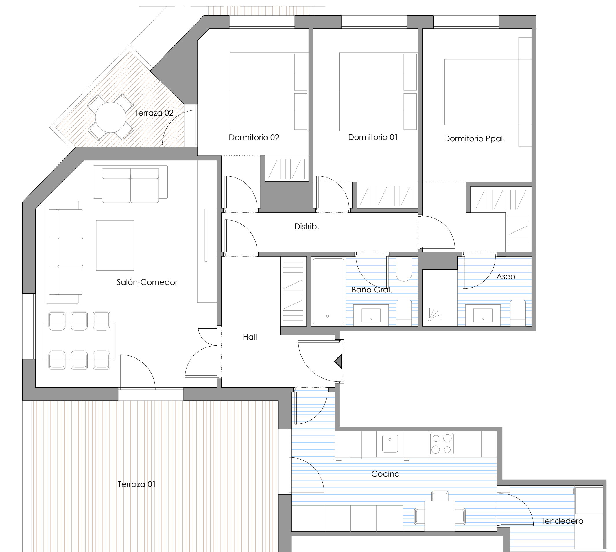
VIVIENDA TIPO-08 3D E: 1/50
